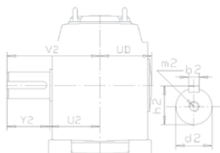
Type D2PSF
